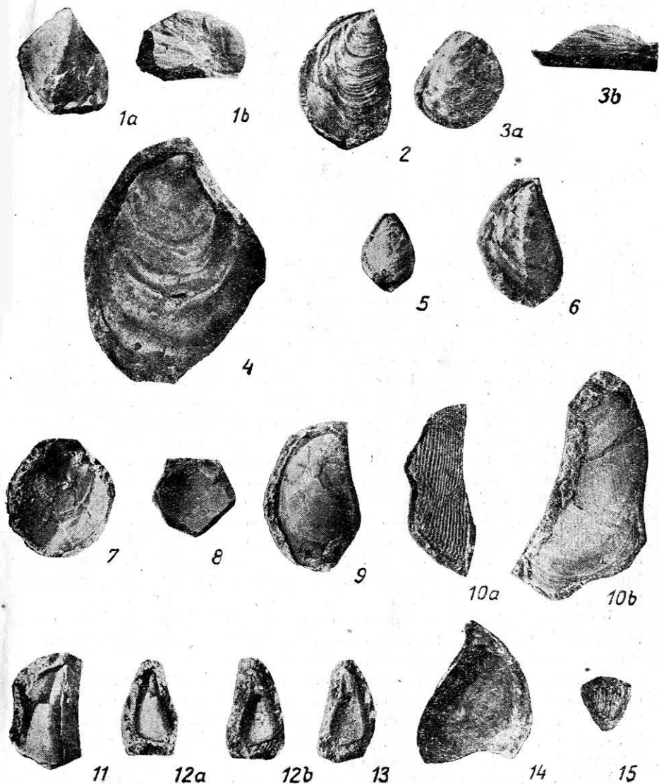
Фиг. 1. Inoceramus cf. concentricus Park., а — левая створка, вид сверху; б — она же сзади. Фиг. 2—6. Inoceramus interruptus Schmidt. 2, 4, 6 — правые створки; 3—5 — левые створки, 3а — сверху, 3б — сзади. Фиг. 7 и 8. Camptonectes striato-punctatus Roem. Отпечатки на породе. Фиг. 9 и 10. Lima longa Roem. 9 — ядро правой и 10б — ядро левой створки, 10а — участок скульптуры (отпечаток на породе). Фиг. 11—13. Pelecypoda gen. et sp. n. inden. 11, 12а — ядра левых створок. 12б, 13 — внутренняя поверхность створок (отпечатки на пластелине). Фиг. 14. Dreissensia sp. Левая створка изнутри. Фиг. 15. Одиночный коралл.
